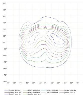
Isocandela(rectangle)
