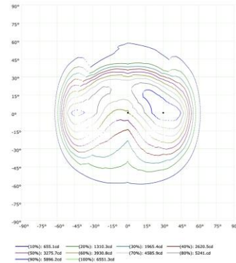
Isocandela(rectangle)
